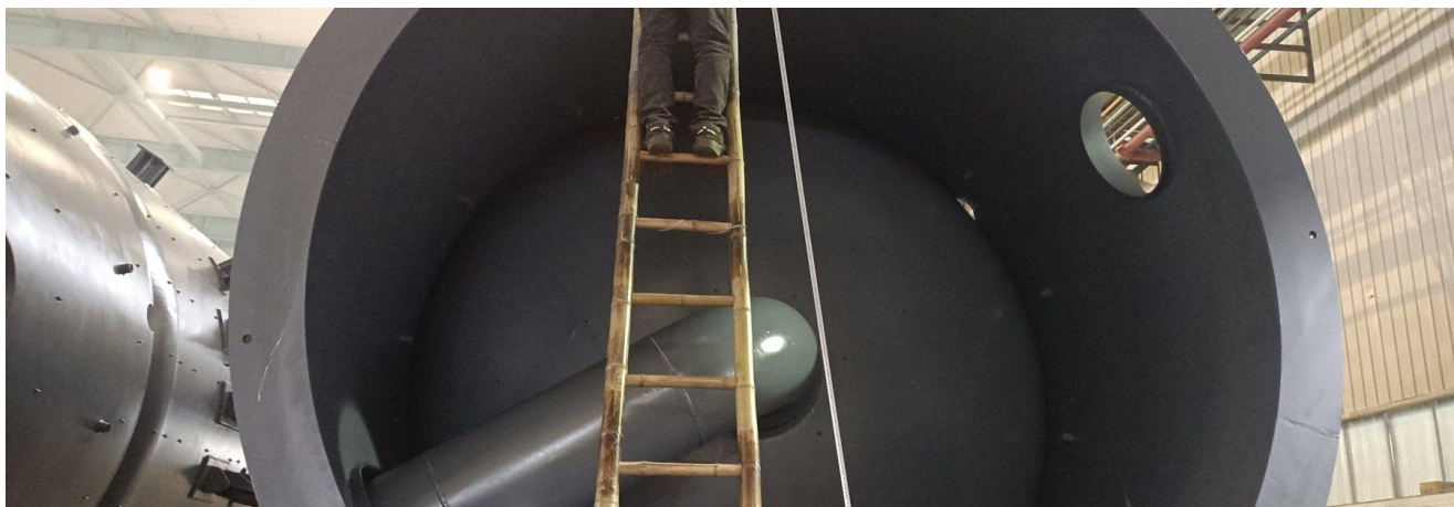
塔器内部：内件检查
